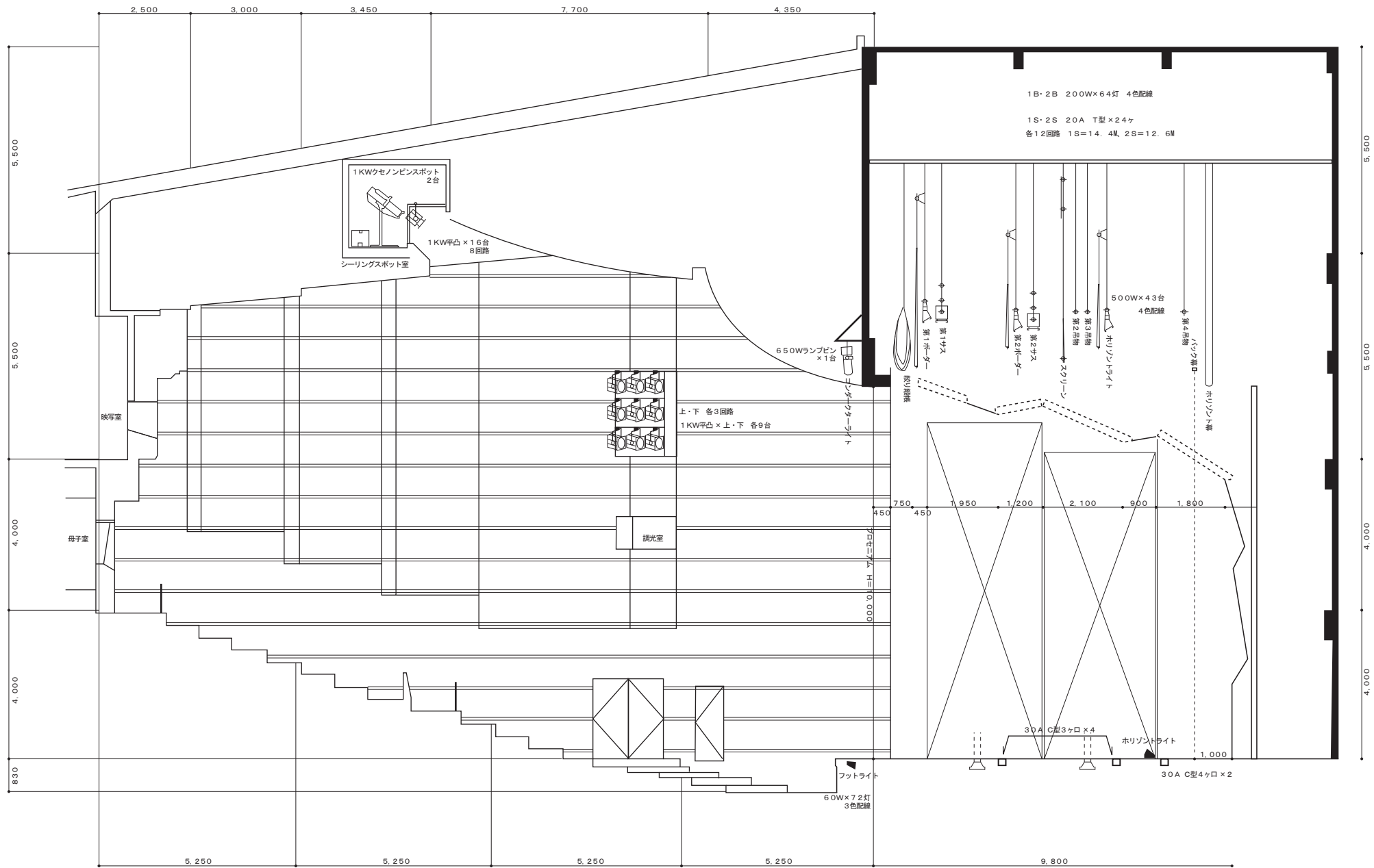
さぬき市志度音楽ホール大ホール断面図
