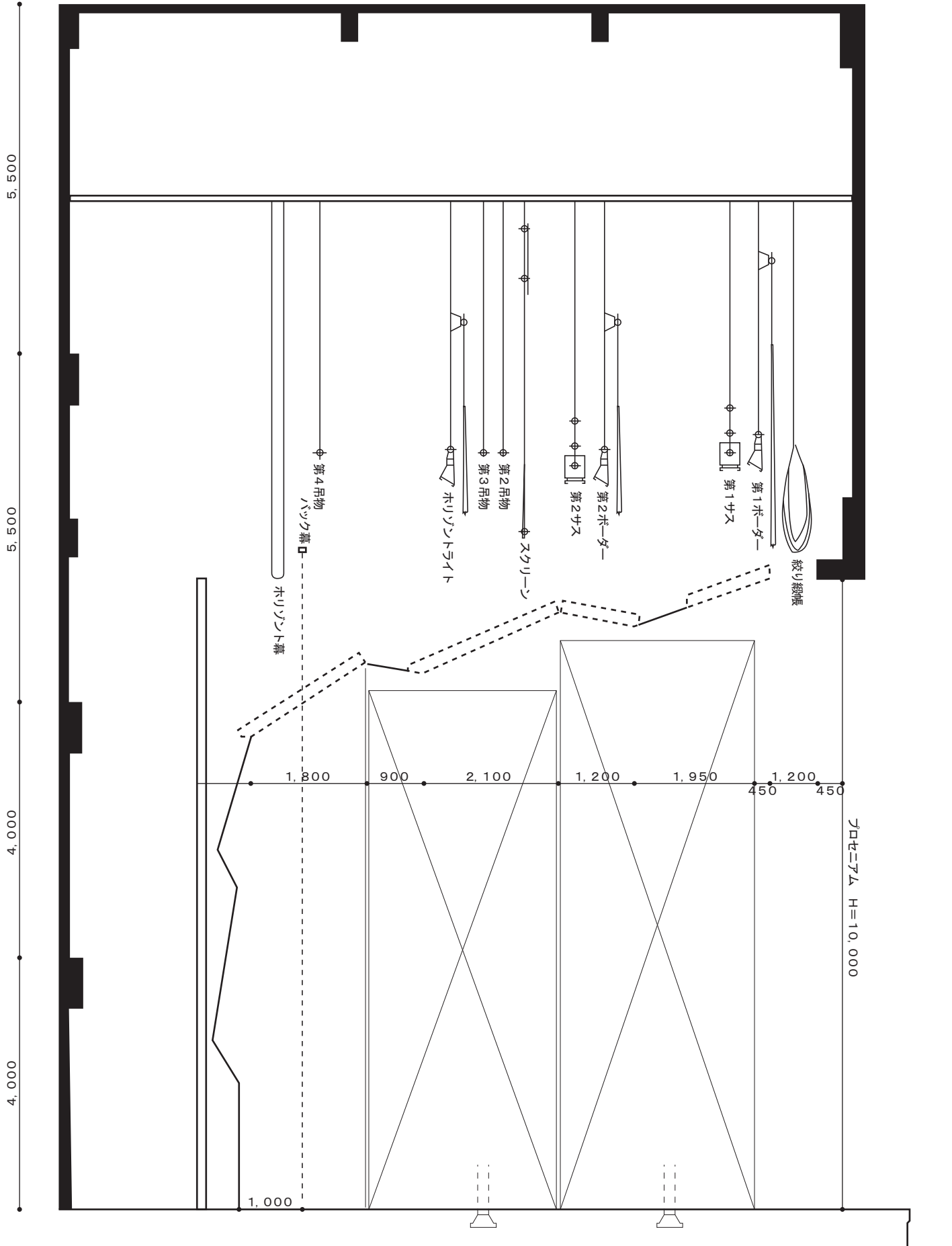
さぬき市志度音楽ホール大ホール舞台断面図
